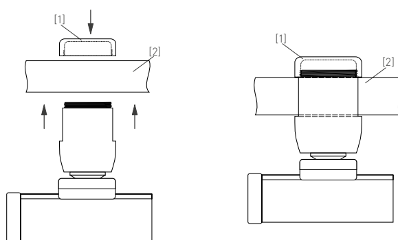
Рис. 2. Установка светильника
