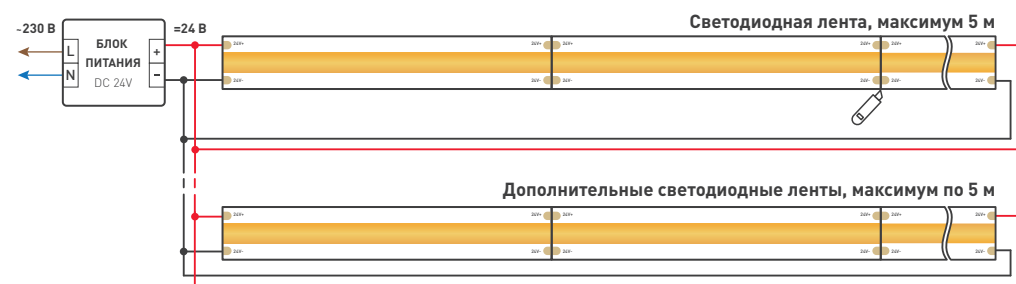
Схема 1. Подключение нескольких светодиодных лент с двух сторон Рекомендуется использовать для обеспечения равномерного свечения ленты по всей длине.
