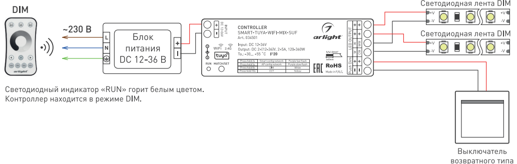
Рисунок 1. Схемы подключения контроллера SMART-TUYA-WIFI-MIX-SUF
