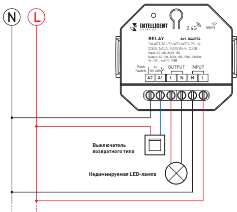
Рис. 1. Схема подключения релейного модуля SMART при помощи выключателя возвратного типа
