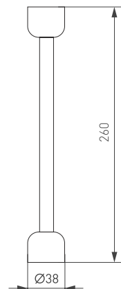
Рис. 1. Чертеж и габаритные размеры
